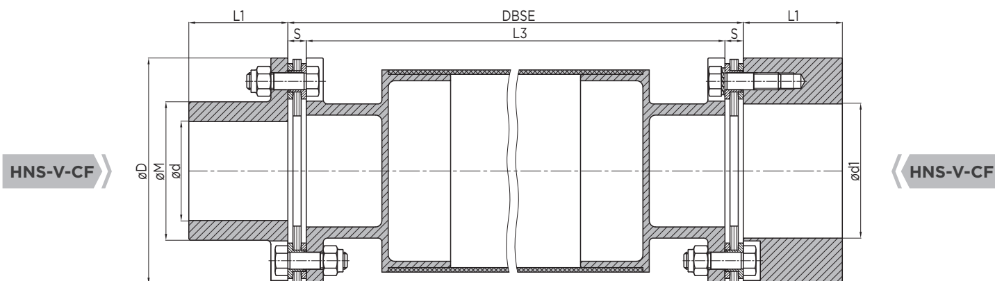
Giunto con un mozzo maggiorato Coupling with large hub
