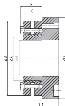
MOZZO MAGGIORATO V Large Hub V
